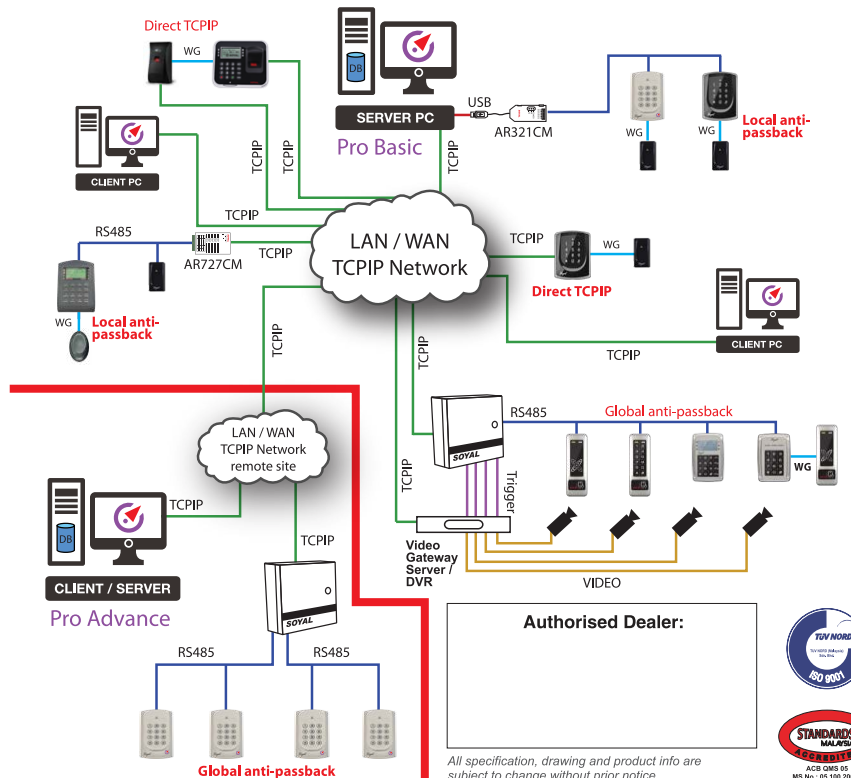
AR716-E18 & AR727i network module
