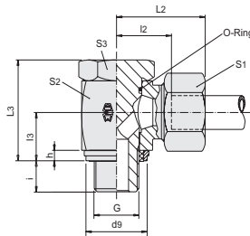
Ausführung mit Dichtring EDE (Innenring aus NBR anvulkanisiert) für Ausdehnung DIN 3852/d4 schmal Model with EDE seal (inner seal made of vulcanized NBR) for narrow DIN 3852/d4 bore Modèle avec bague d'étanchéité EDE (Bague intérieure en NBR vulcanisé) pour alésage DIN 3852/d4 étroit
