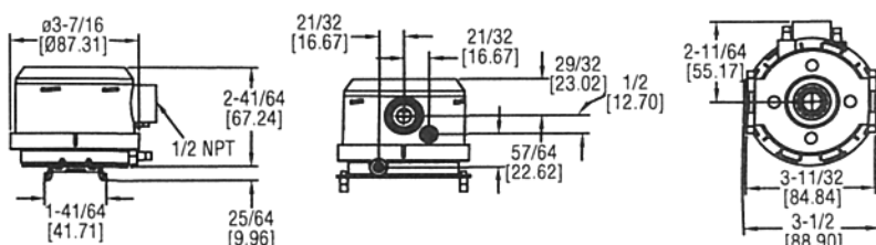
DIN Mount Bracket
