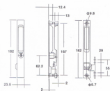
Dimension of A5 & A6
