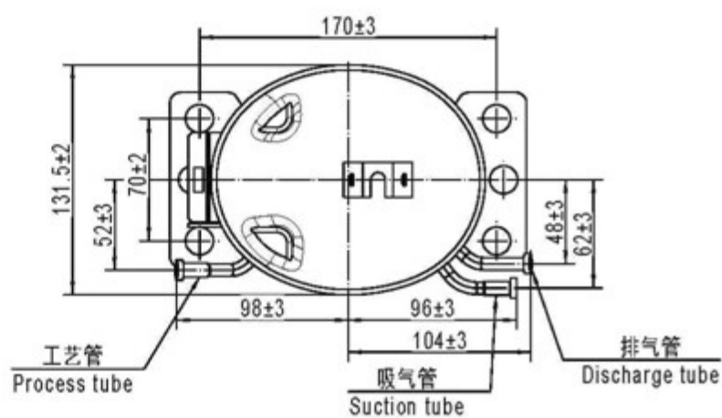
Y 系列外观 Y Series External Views
