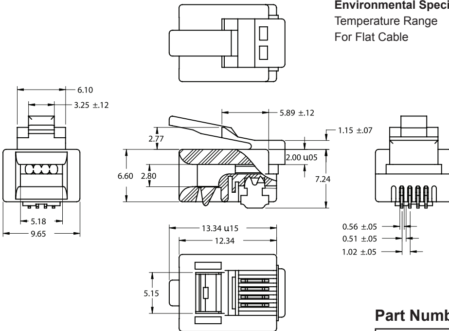
Dimensions : Millimetres
