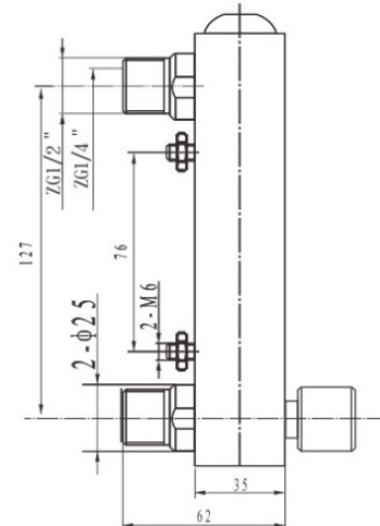
LZT-10□□M-V
