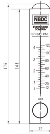
LZT-10A□□M-V LZT-10T□□M-V
