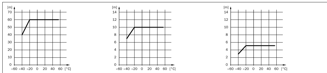
Fig. 9: L41X-33MA2A
