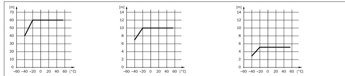
Fig. 9: L41X-33MA2A
