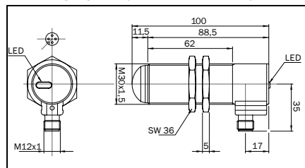
Fig. 5: L41X-33MA2A
