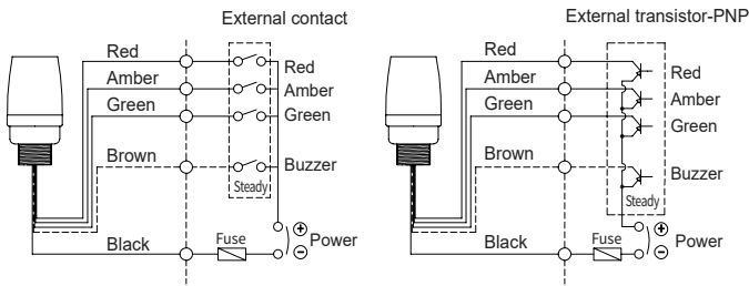
EMCL50U, EMCL50U-BZ
