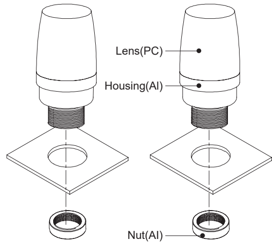
EMCL50U, EMCL50U-BZ
