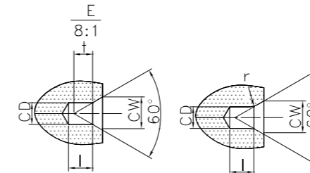
A型中心定位孔
