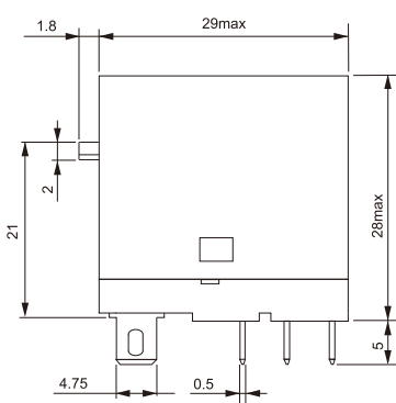
DRPT-1C
