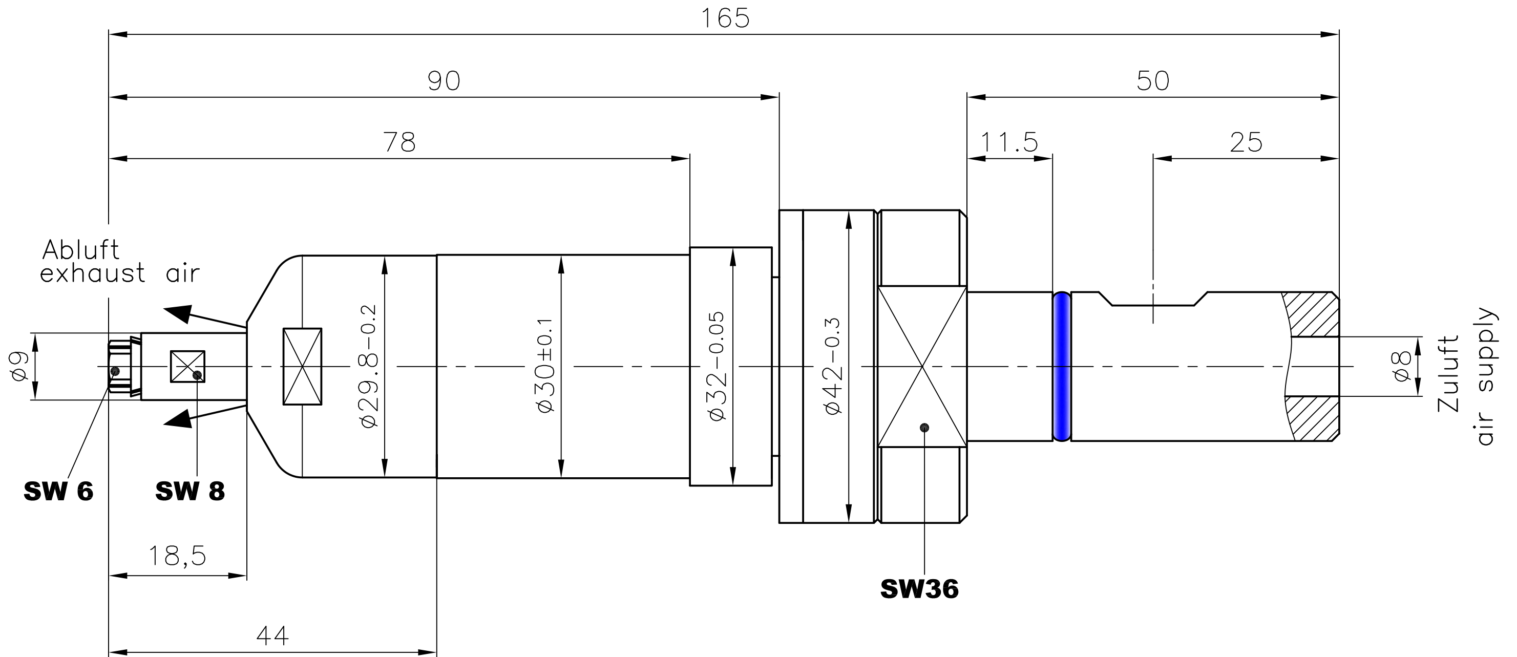
Roboterspindel ESK1000 W20 60019587
