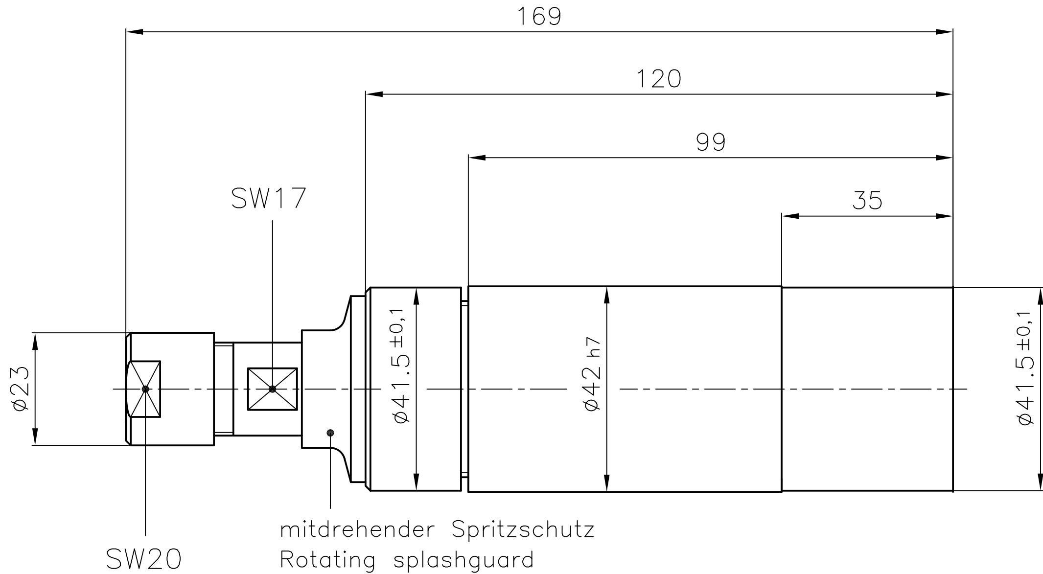
Einbaubohrmotor EBM 19000 SL 29946527
