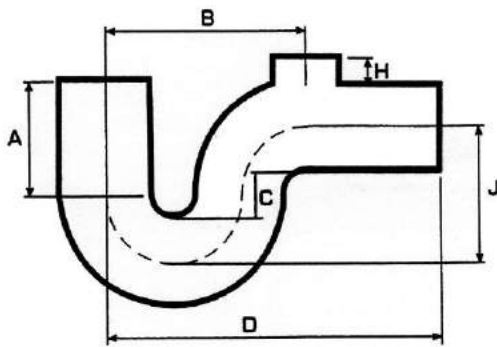
4 x 4 x 2 'P' Trap
