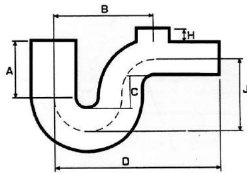
4 x 3 x 2 'P' Trap
