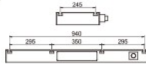
EEPМ-30100SL
