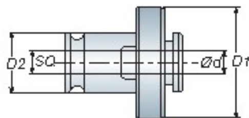
剛性絲攻筒夾 - FIG.2
