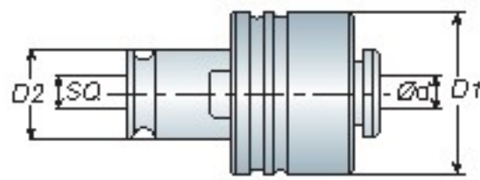
扭力絲攻筒夾 - FIG.1
