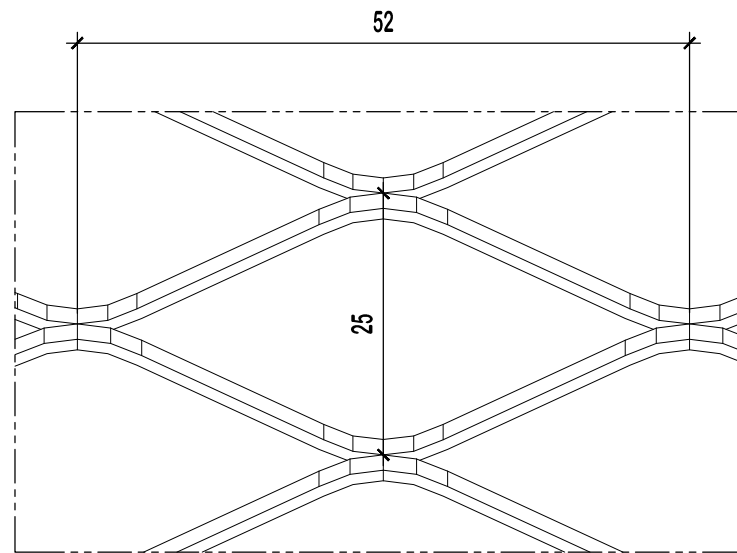
05 DETAIL A SCALE - N.T.S
