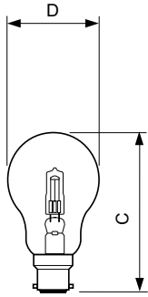
HalClass 28W B22 240V A55 CL
