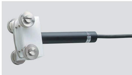
●SK-S402K 回転表面用 (ローラ型) 0~300°C 25×50×25mm 取っ手部φ15×L90mm コード1.1m付 ¥22,500 (税抜き) (センサ精度 クラス2)
