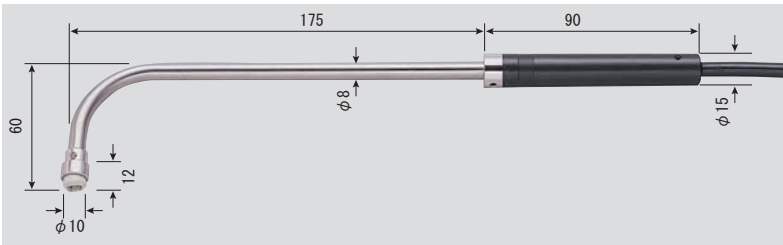
●SK-S303K 静止表面用L型 (中・高温用) 0~800°C 先端部φ10×L12mm コード1.1m付 No. 8080-54 ¥13,000 (税抜き) (センサ精度 クラス2)
