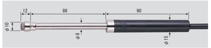
●SK-S306K 静止表面用 (低温) -30~250°C 先端部φ10×L12mm コード1.1m付 No. 8080-60 ¥13,000 (税抜き) (センサ精度 クラス2)
