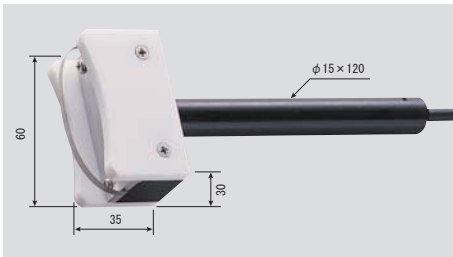
●SK-S401K 曲面表面用 (パイプ等) 0~250°C 先端部30×35×60mm コード1.1m付 No. 8080-70 ¥16,500 (税抜き) (センサ精度 クラス2)
