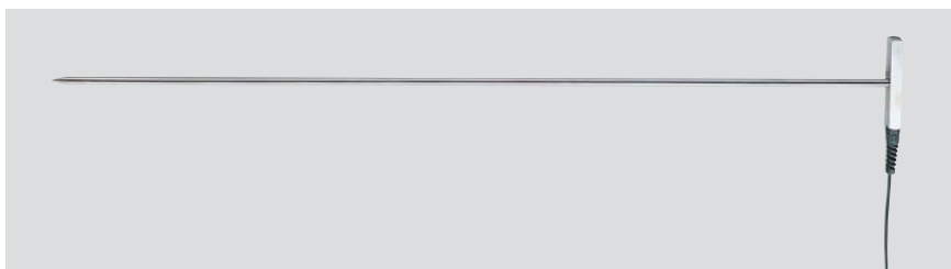
●SK-S108K 堆肥用センサ 0~300°C φ8×L900mm (材質:SUS304) コード1.1m付 No. 8080-38 ¥17,500 (税抜き) (センサ精度 クラス2)
