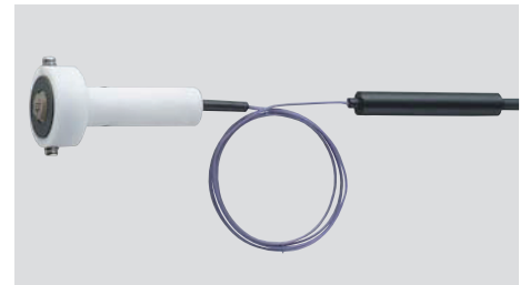
●SK-S403K 静止表面用 (マグネット型) 0~200°C 先端部φ30×R12mm 取っ手部φ15×L50mm コード1.1m付 ¥19,500 (税抜き) (センサ精度 クラス2)
