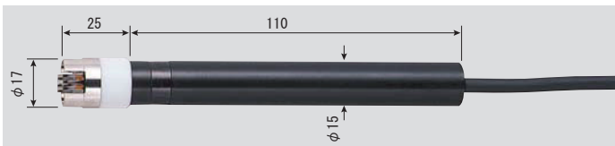
●SK-S307K 静止表面用 (一般計測、低温) -30~400°C 先端部φ17×L25mm コード1.1m付 No. 8080-62 ¥13,000 (税抜き) (センサ精度 クラス2)
