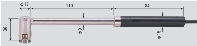
●SK-S305K 静止表面用 (90° 角度可変、中温) -30~500°C 先端部φ17×L36mm コード1.1m付 No. 8080-58 ¥19,500 (税抜き) (センサ精度 クラス2) (写真は90°に曲げた状態)
