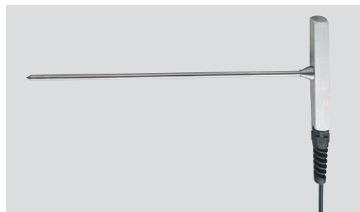
●SK-S109K アスファルト用センサ 0~300°C φ5×L250mm (材質:SUS304) コード1.1m付 No. 8080-40 ¥15,000 (税抜き) (センサ精度 クラス2)
