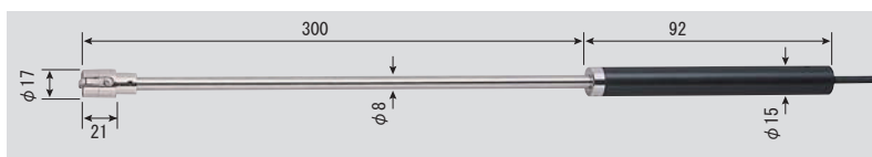
●SK-S302K 静止表面用 (ロングサイズ) 0~600°C 先端部φ17×L21mm コード1.1m付 No. 8080-52 ¥20,500 (税抜き) (センサ精度 クラス2)
