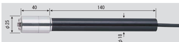
●SK-S301K 静止表面用 (中温) 0~600°C 先端部φ25×L40mm コード1.1m付 No. 8080-50 ¥14,000 (税抜き) (センサ精度 クラス2)
