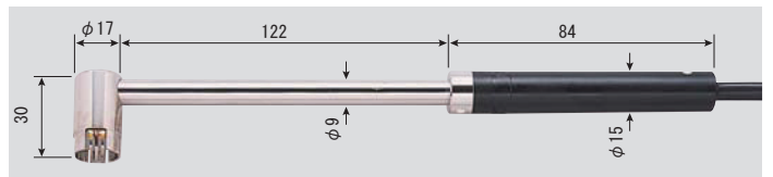
●SK-S308K 静止表面用 (L型センサ、中温) -30~600°C 先端部φ17×L30mm コード1.1m付 No. 8080-64 ¥15,000 (税抜き) (センサ精度 クラス2)
