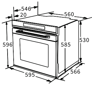
OVEN / FV-EL63
