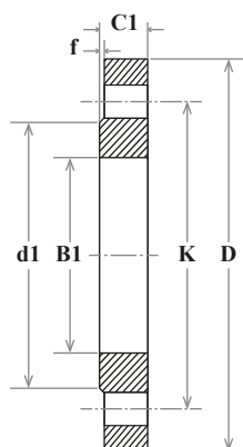
SECTION A-A TYPE 01
