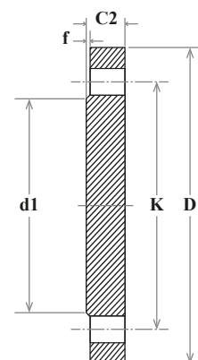
SECTION A-A TYPE 05
