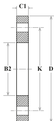
SECTION A-A TYPE 02
