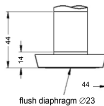
dairy pipe DN25 DIN 11851 (P_N \geq 0.25 bar)
