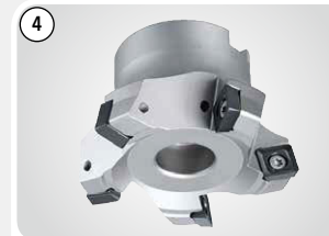
Hochgeschwindigkeits-Planfräsen High feed face milling
