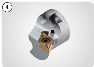
Schlichten Innenkontur Finishing
