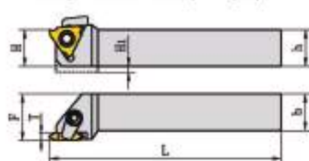
形式 I Type I
