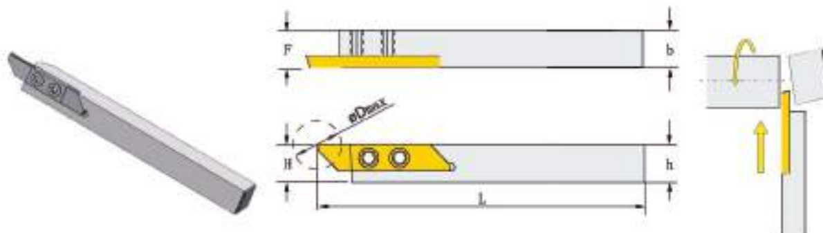
图为右手刀具
