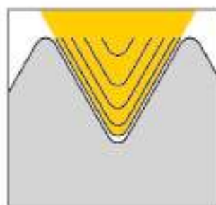
切屑面积 + 跳跃走刀
