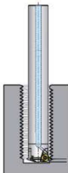
A型适用于小螺距以及退刀槽较短的情况 for short pitches
