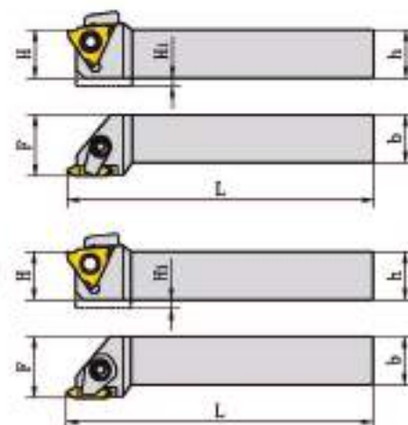
形式 I Type I
