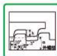
标准 美制API螺纹 STD. 5B:1979
