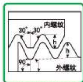
标准 美制API螺纹 SPEC. 7:1990 公差等级标准 美制API螺纹
