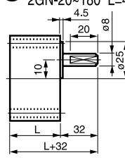
② 2GN-3~18 L=32 重量 0.35kg 2GN-20~180 L=42 重量 0.45kg
