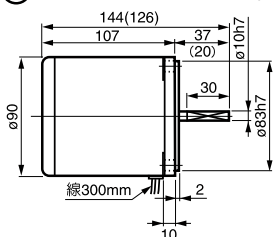
⑩ 5IK40A(GN)-口 重量 2.5kg
