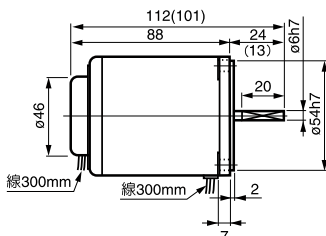
① M206-口 重量 0.9kg
