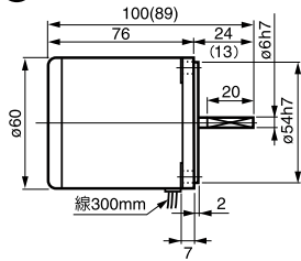
① 2IK6A(GN)-口 重量 0.7kg
