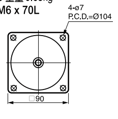
⑱ 5GU-10XKS 重量 0.65kg 適用螺絲: M6 x 70L
