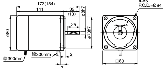
⑦ 4IK25A(GN)-□B 重量 2kg
