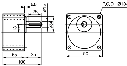
⑭ 5GU-3~180KB 重量 1.3kg (60, 90, 120, 150W 共用)
