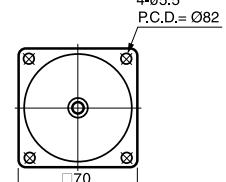
⑥ 3GN-10X 重量 0.35kg
