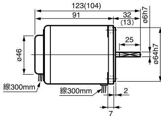
④ M315-口 重量 1.3kg
