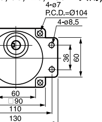
⑰ 5GU-3~180K 重量 1.3kg (60, 90, 120, 150W 共用)
