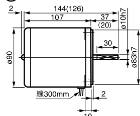
⑩ 5RK40A(GN)-□ 重量 2.5kg
