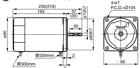
⑬ M560-□B 重量 3.1kg
