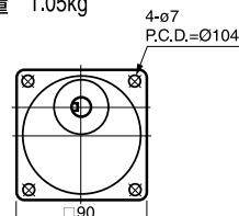
⑪ 5GN-3~18 L=42 重量 0.7kg (40~120W 共用) 5GN-20~180 L=58 重量 1.05kg
