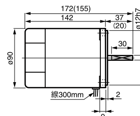
⑬ 5RK60 GN-□ 重量 2.6kg
