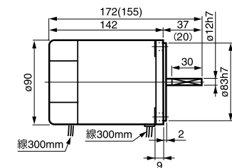
⑬ M560-口 重量 2.7kg
