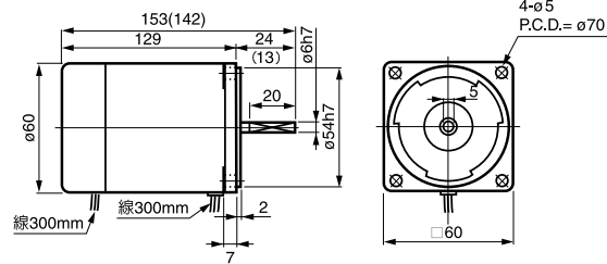
① 2IK6A(GN)-□B 重量 1.2kg
