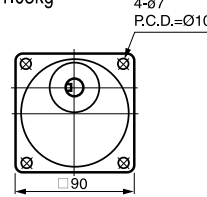
⑪ 5GN-3~18 L=42 重量 0.7kg (40~150W 共用) 5GN-20~180 L=58 重量 1.05kg
