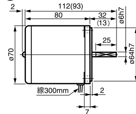
④ 3RK15A(GN)-□ 重量 1.2kg
