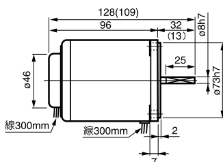
⑦ M425-口 重量 1.8kg
