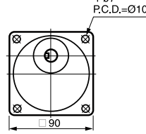
⑭ 5GU-3~180KB 重量 1.3kg (60, 90, 120, 150W 共用)
