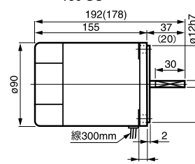
⑯ 5RK 120 GN-□ 重量 3.4kg
