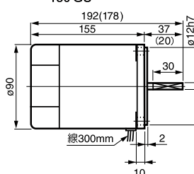
⑯ 5IK 120 GN-口 重量 3.4kg 150 GU
