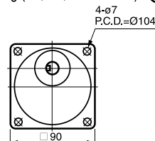
⑭ 5GU-3~180 KB 重量 1.3kg (60, 90, 120W 共用)
