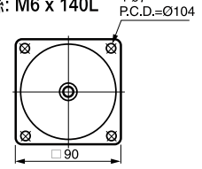
⑮ 5GU-10XK 重量 0.65kg 適用螺絲: M6 x 140L
