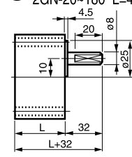
② 2GN-3-18 L=32 重量 0.35kg 2GN-20-180 L=42 重量 0.45kg
