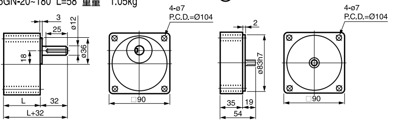
⑪ 5GN-3-18 L=42 重量 0.7kg (40~120W 共用) 5GN-20-180 L=58 重量 1.05kg
