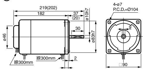
⑩ M540-□B 重量 3kg
