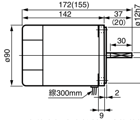
⑯ 5IK 120 GN-口 重量 3.4kg 150 GU
