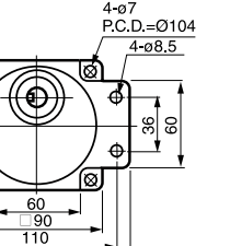
⑰ 5GU-3-180 K 重量 1.3kg (60, 90, 120, 150W 共用)
