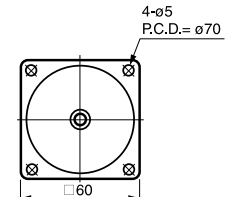
③ 2GN-10X 重量 0.3kg
