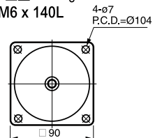
⑮ 5GU-10XK 重量 0.65kg 適用螺絲: M6 x 140L
