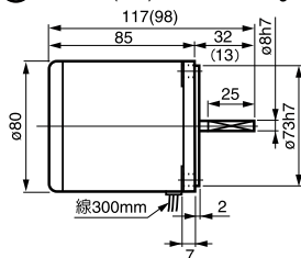
⑦ 4IK25A(GN)-口 重量 1.6kg
