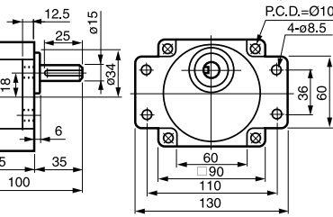
⑰ 5GU-3~180K 重量 1.3kg (60, 90, 120W 共用)
