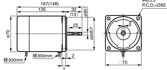
④ 3IK15A(GN)-□B 重量 1.6kg
