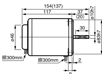
⑩ M540-口 重量 2.6kg
