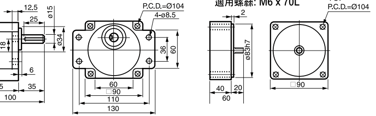
⑰ 5GU-3~180K 重量 1.3kg (60, 90, 120W 共用)
