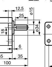
⑰ 5GU-3~180K 重量 1.3kg (60, 90, 120, 150W 共用)
