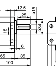
⑰ 5GU-3-180 K 重量 1.3kg (60, 90, 120, 150W 共用)
