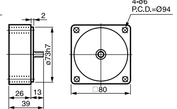
⑨ 4GN-10X 重量 0.45kg
