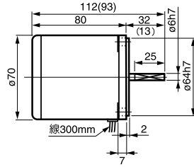
④ 3IK15A(GN)-口 重量 1.1kg
