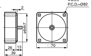
⑥ 3GN-10X 重量 0.35kg
