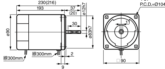
⑬ 5IK60 GN - □ GU 重量 3.1kg
