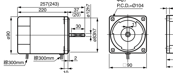
⑯ 5IK 120 GN - □ 150 GU 重量 4kg
