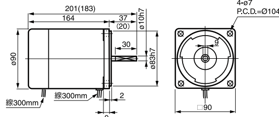
⑩ 5IK40A(GN)-□B 重量 3kg
