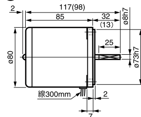
⑦ 4RK25A(GN)-□ 重量 1.65kg
