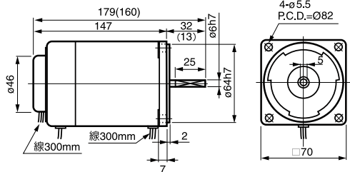
④ M315-□B 重量 1.1kg
