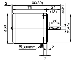
① 2RK6A(GN)-□ 重量 0.8kg
