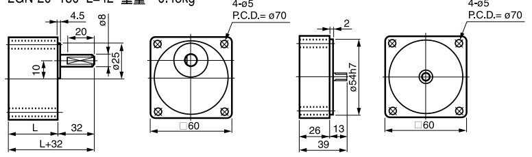
② 2GN-3-18 L=32 重量 0.35kg 2GN-20-180 L=42 重量 0.45kg
