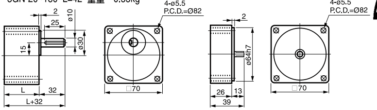
⑤ 3GN-3-18 L=32 重量 0.45kg 3GN-20-180 L=42 重量 0.55kg
