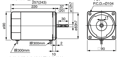
⑯ M590-□B 重量 4kg M5120-□B
