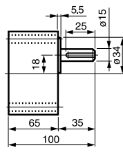
⑭ 5GU-3~180KB 重量 1.3kg (60, 90, 120, 150W 共用)
