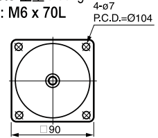
⑱ 5GU-10XKS 重量 0.65kg 適用螺絲: M6 x 70L
