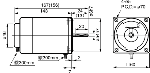
① M206-□B 重量 1.2kg
