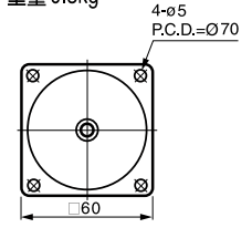
③ 2GN-10X 重量 0.3kg
