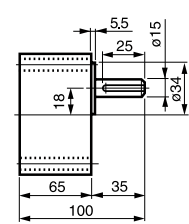
⑭ 5GU-3-180 KB 重量 1.3kg (60, 90, 120, 150W 共用)
