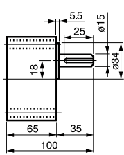
⑭ 5GU-3~180 KB 重量 1.3kg (60, 90, 120W 共用)
