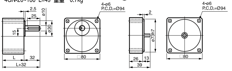
⑧ 4GN-3-18 L=35.5 重量 0.5kg 4GN-20-180 L=49 重量 0.7kg
