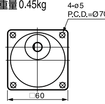
② 2GN-3~18 L=32 重量 0.35kg 2GN-20~180 L=42 重量 0.45kg
