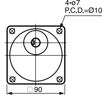
⑭ 5GU-3-180 KB 重量 1.3kg (60, 90, 120, 150W 共用)
