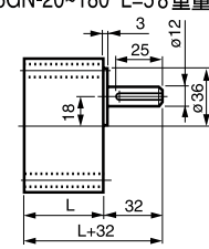
⑪ 5GN-3-18 L=42 重量 0.7kg (40~150W 共用) 5GN-20-180 L=58 重量 1.05kg
