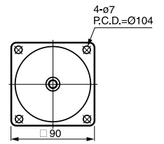
⑨ 5GU-10XK 重量 0.65kg 適用螺絲: M6 x 140L
