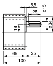
⑭ 5GU-3~180KB 重量 1.3kg (60, 90, 120, 150W 共用)
