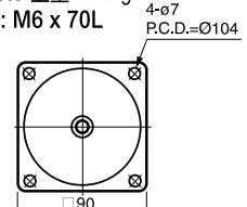
⑱ 5GU-10XKS 重量 0.65kg 適用螺絲: M6 x 70L
