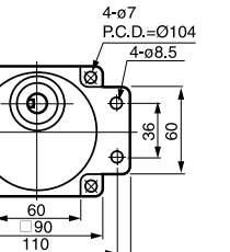
⑪ 5GU-3~180K 重量 1.3kg (60, 90, 120, 150W 共用)
