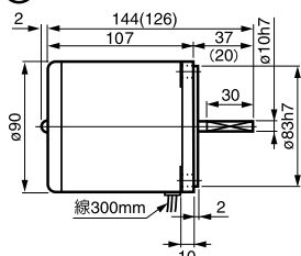
⑩ 5RK40A(GN)-口 重量 2.5kg
