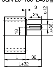
⑪ 5GN-3~18 L=42 重量 0.7kg (40~150W 共用) 5GN-20~180 L=58 重量 1.05kg
