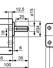
⑪ 5GU-3~180K 重量 1.3kg (60, 90, 120, 150W 共用)
