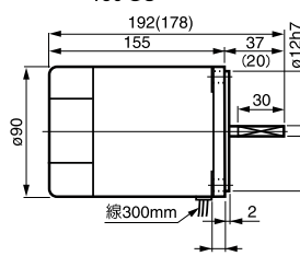
⑯ 5RK 90 A GN-口 重量 3.4kg 120 GN 150 GU
