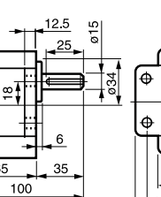
⑰ 5GU-3-180 K 重量 1.3kg (60, 90, 120, 150W 共用)
