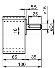
⑭ 5GU-3~180 KB 重量 1.3kg (60, 90, 120W 共用)
