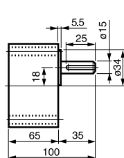
⑧ 5GU-3~180KB 重量 1.3kg (60, 90, 120, 150W 共用)
