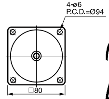
③ 4GN-10X 重量 0.45kg
