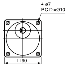
⑧ 5GU-3~180KB 重量 1.3kg (60, 90, 120, 150W 共用)
