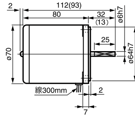
④ 3RK15A(GN)-口 重量 1.2kg
