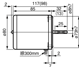
⑦ 4RK25A(GN)-口 重量 1.65kg
