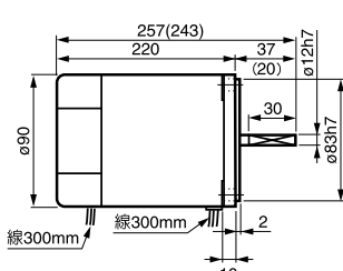
⑩ 5IK120 GN -□B / 5IK150 GN -□B GU 重量 3.1kg
