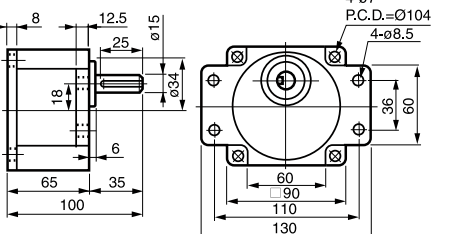
⑰ 5GU-3~180K 重量 1.3kg (60, 90, 120, 150W 共用)
