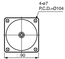
⑥ 5GN-10X 重量 0.6kg
