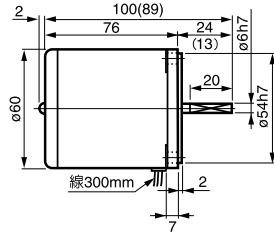
① 2RK6A(GN)-口 重量 0.8kg
