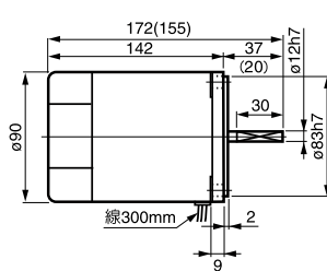
⑦ 5IK60 GN-□ / 5IK90 GN-□ 重量 2.6kg A GU / A GU
