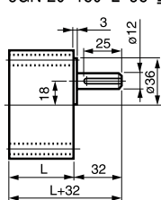
⑪ 5GN-3~18 L=42 重量 0.7kg (40~120W 共用) 5GN-20~180 L=58 重量 1.05kg
