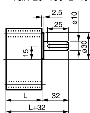
⑧ 4GN-3~18 L=35.5 重量 0.5kg 4GN-20~180 L=49 重量 0.7kg
