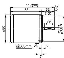
① 4IK25A(GN)-□ 重量 1.6kg
