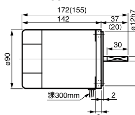
⑬ 5RK60 GN-口 重量 2.6kg
