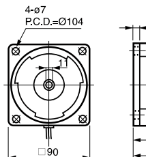
⑩ 5IK120 GN -□B / 5IK150 GN -□B GU 重量 3.1kg
