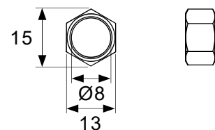
Nut
