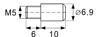
Optional : Extension Pin
