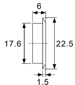
Rosette
