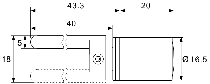
Rosette
