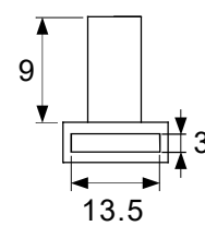
S-Nut (Peg)
