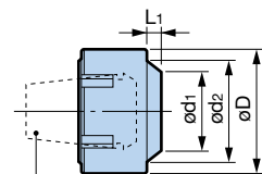
New Baby Collet (NBC)
