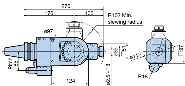
Fig. 1 Max. 6.000min -1
