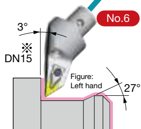
S50-DDJNR-33075-15 -DDJNL-33075-15
