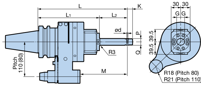
Fig. 2 Max. 2,000min -1
