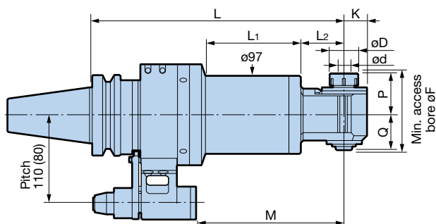
Fig. 2 Max.6,000min -1
