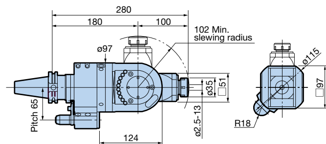
Fig. 1 Max. 6,000min -1
