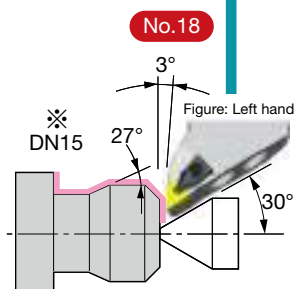
F63-DDJNR-45055-15 -DDJNL-45055-15
