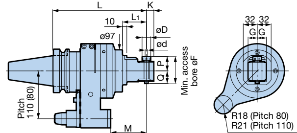
Fig. 1 Max.6,000min -1
