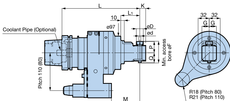
Fig. 1 Max.6,000min -1
