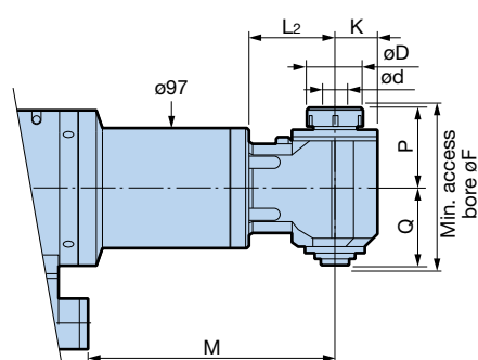
Fig. 3 Max.3,000min -1
