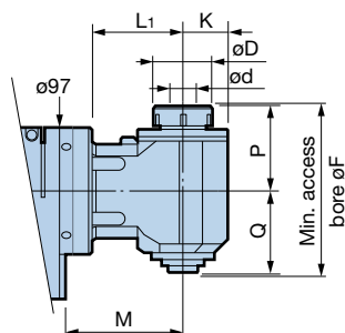
Fig. 3 Max.3,000min -1
