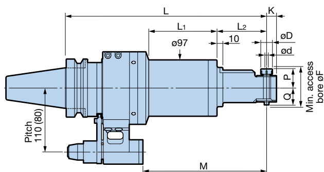
Fig. 1 Max.6,000min -1
