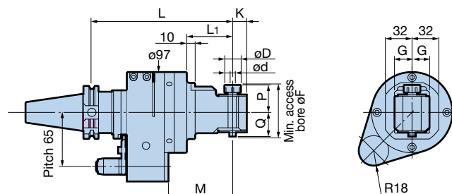
Fig. 1 Max. 6,000min -1
