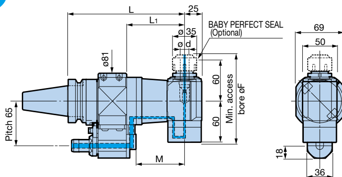
Fig. 1 Max.5,000min -1
